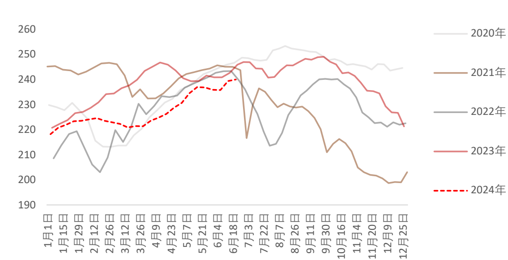
247家钢厂日均铁水产量（万吨）
